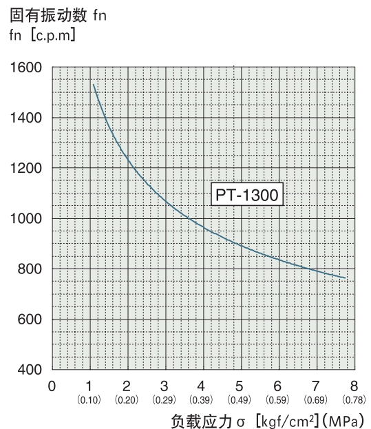
●图2 固有振动数~应力特性
