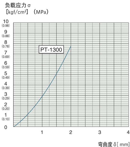
●图1 应力~弯曲特性
